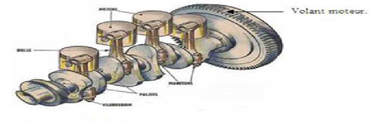
Figure I.11 : le volant moteur.
