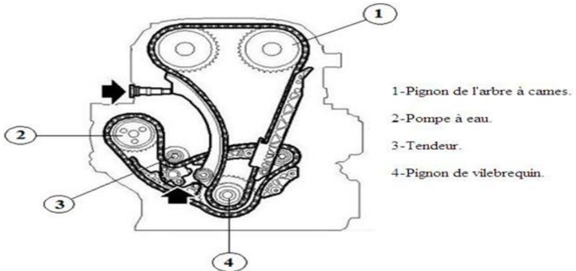
Figure I.13 : la chaîne de distribution.
