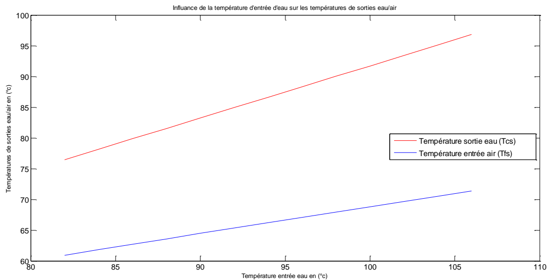
Figure III.18 : Evolution des températures de sortie d'eau et d'air en fonction de la température entrée eau pour ( T_{fe}=45^{\circ}\text{C} , m_e=45\text{kg/s} , m_a=6.52\text{kg/s} ).
