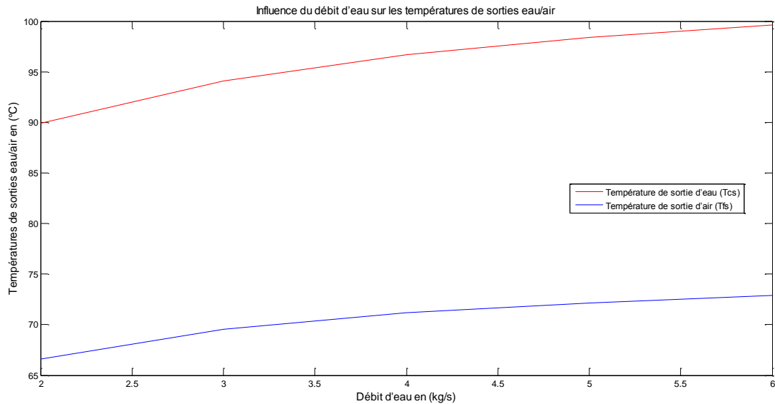
Figure III.16 : Evolution des températures d'eau et d'air en fonction de débit d'eau pour ( T_{ce}=107^{\circ}\text{c} , T_{fe}=45^{\circ}\text{c} , m_a=6.52\text{kg/s} ).
