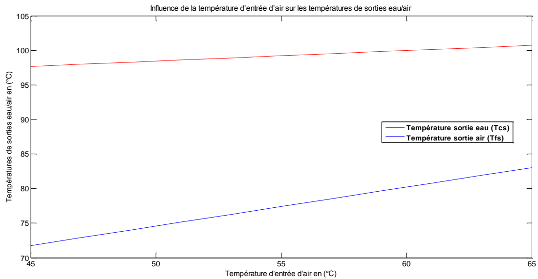
Figure III.18 : Evolution des températures de sortie d'eau et d'air en fonction de la température entrée air pour ( T_{ce}=107^{\circ}\text{C} , m_e=4.54\text{kg/s} , m_a=6.52\text{kg/s} ).
