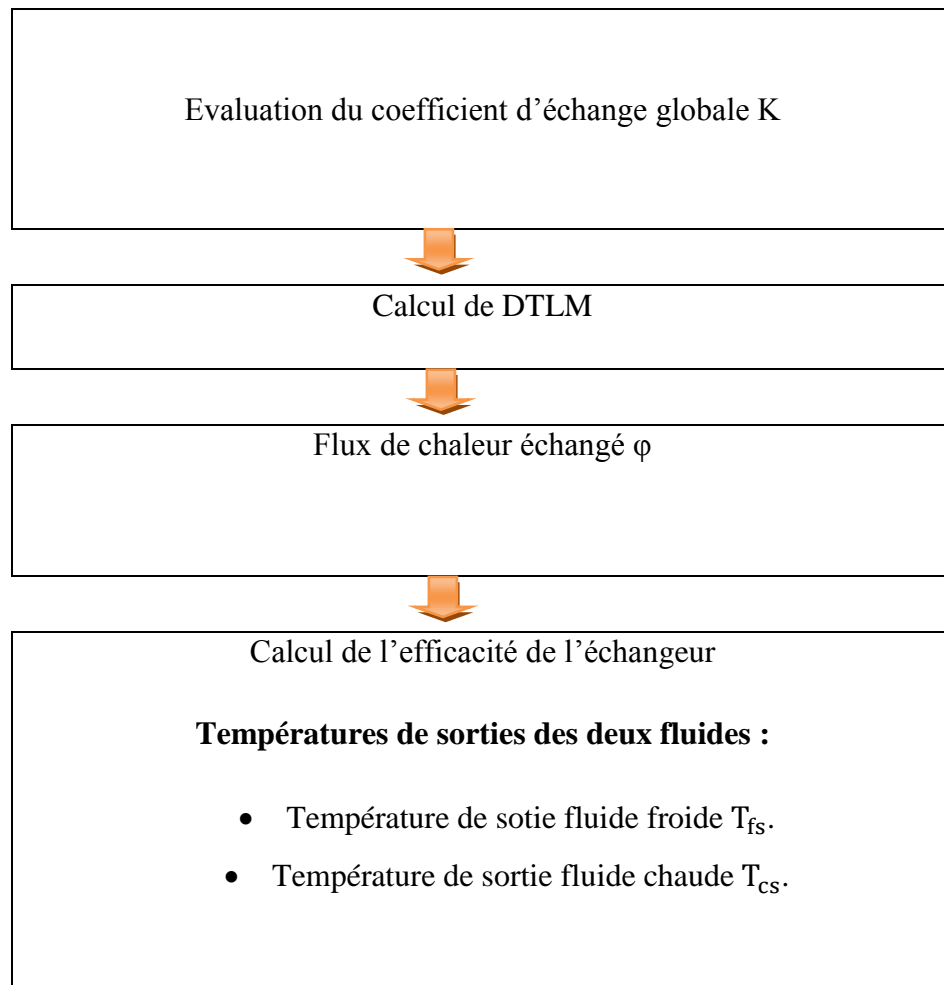
FigureIII.11 :Algorithme de calcul avec la methode de DTLM
