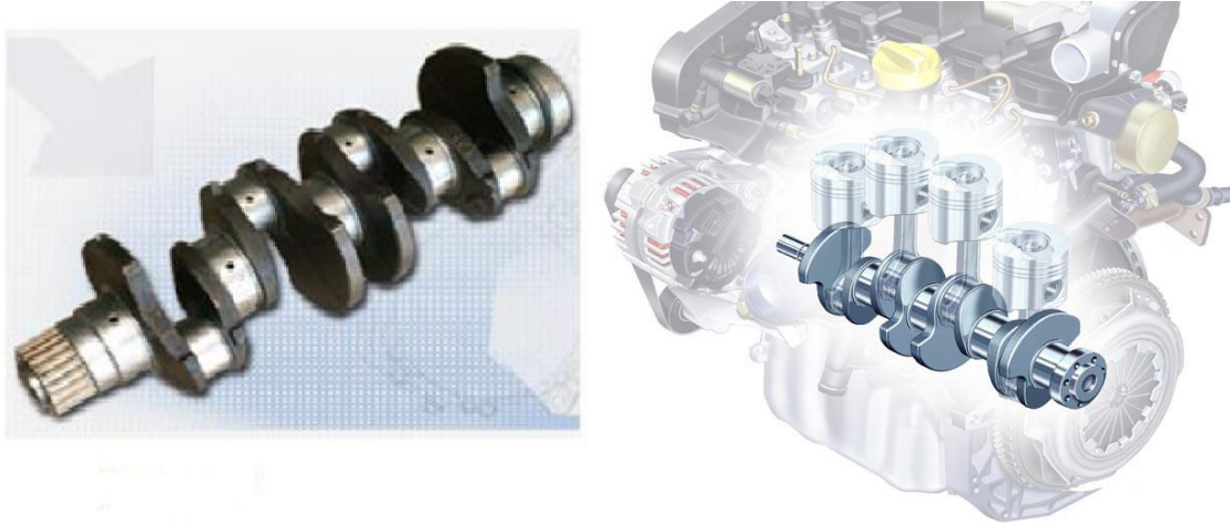
Figure I.8 : le Vilebrequin.
