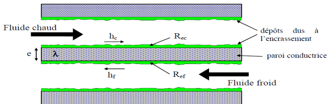
Figure III-7 :l'encrassement dans un échangeur.
