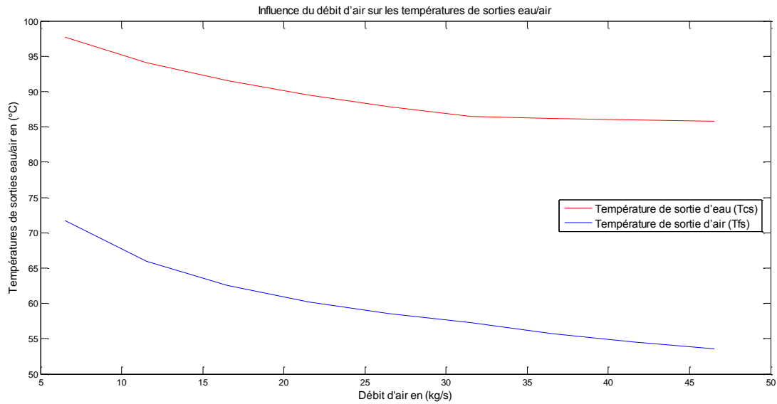
Figure III.17 : Evolution des températures de sorties d'eau et d'air en fonction de débit d'air, Pour ( T_{ce}=107^{\circ}\text{C} , T_{fe}=45^{\circ}\text{C} , m_e=4.54\text{kg/s} )
