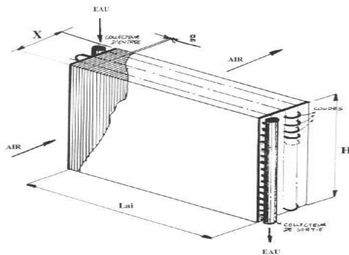
Figure III.9 : Schéma descriptif d'un échangeur à courant croiséé
