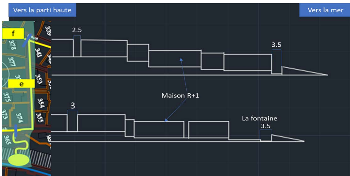
Figure62: coupe du tronçon E source : l'auteur.
