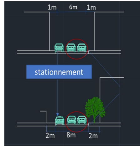
Figure50 : coupe schématique perpendiculaire de la RN24 Source :PPMVS
