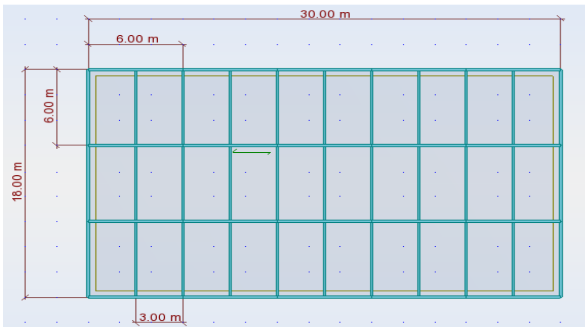
Figure 5.3 différents dimension de la structure dans les deux sens
