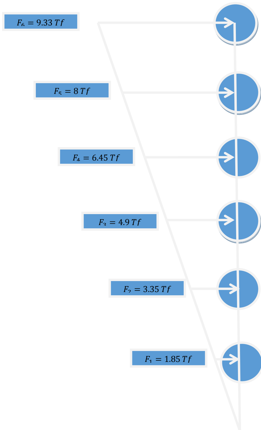
Figure 3.1 Distribution de l'effort tranchant pour chaque étage
