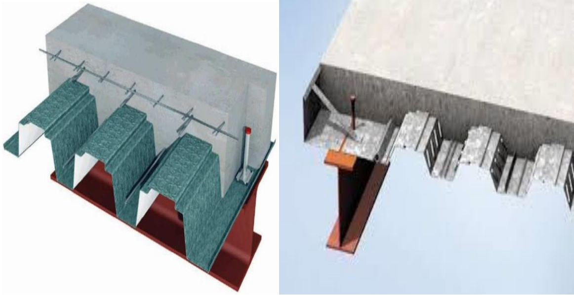
Figure1.7 : plancher collaborant mixte acier (tôle) + béton
