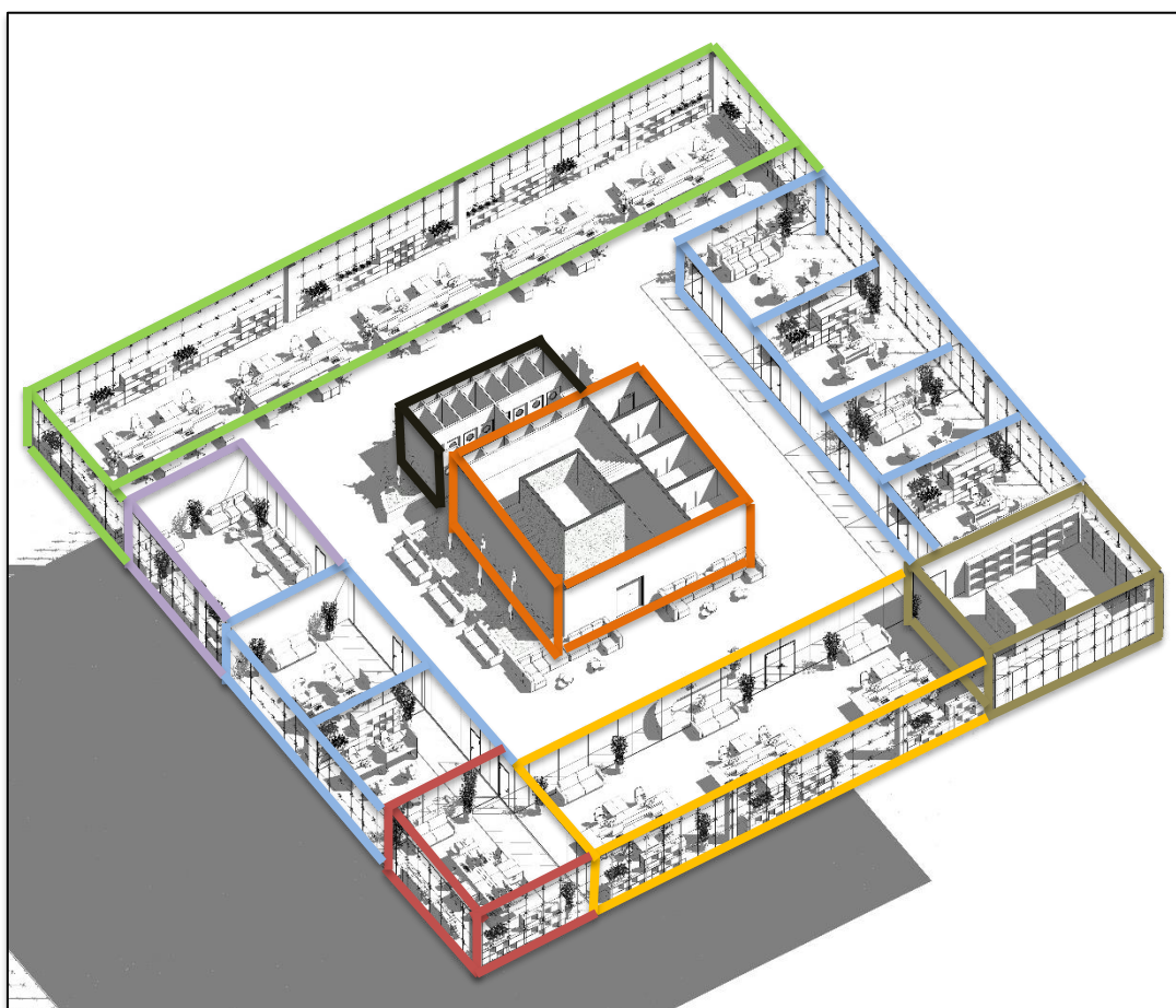
Figure 173 : Élévation 3D de l'étage courant de l'entité archive Source : Revit
