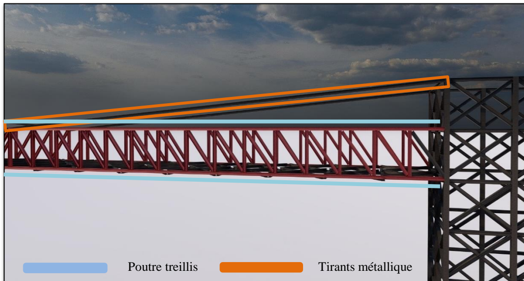
Figure 228 : Structure de la passerelle urbaine du projet . Source : Auteur
