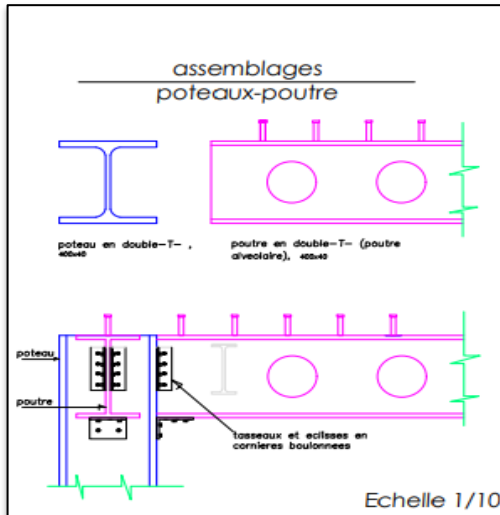
Figure 203 : détail assemblage poutre-poteau. Source : Autocad
