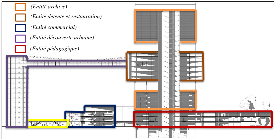
Figure 170 : Coupe illustrant les entités du projet Source : Revit
