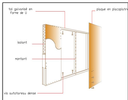
Figure 248 : Détail de la cloison en placo plâtre.
