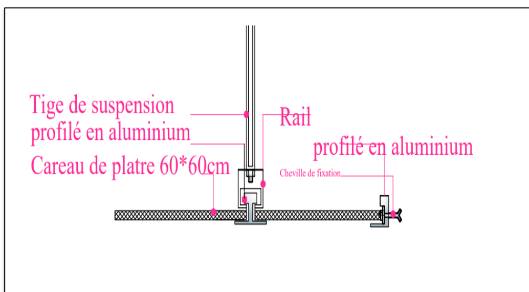
Figure 239 : Détail du faux plafond.
