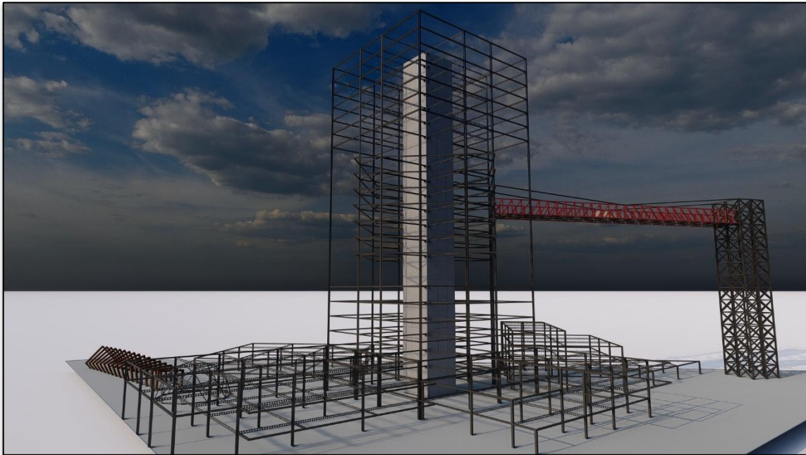
Figure 182: Modélisation 3D de la Structure métallique du projet Source : Auteurs
