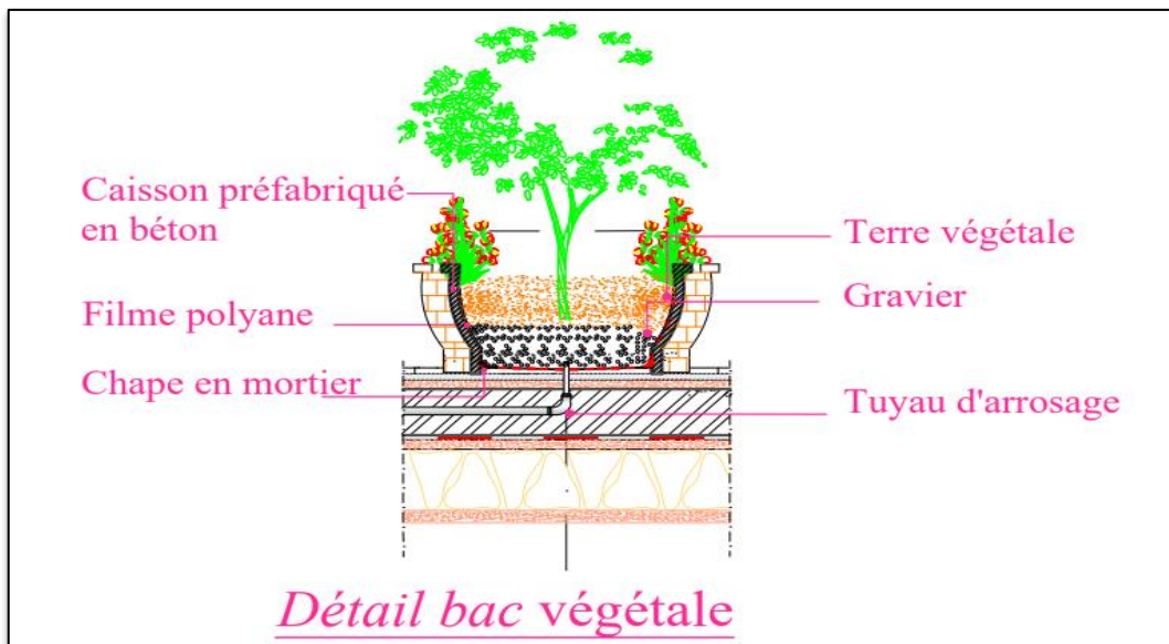
Figure 251 : Détail bac végétale.
