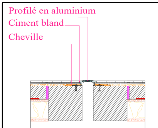
Figure 190 : détail couvre - joint de dilatation
