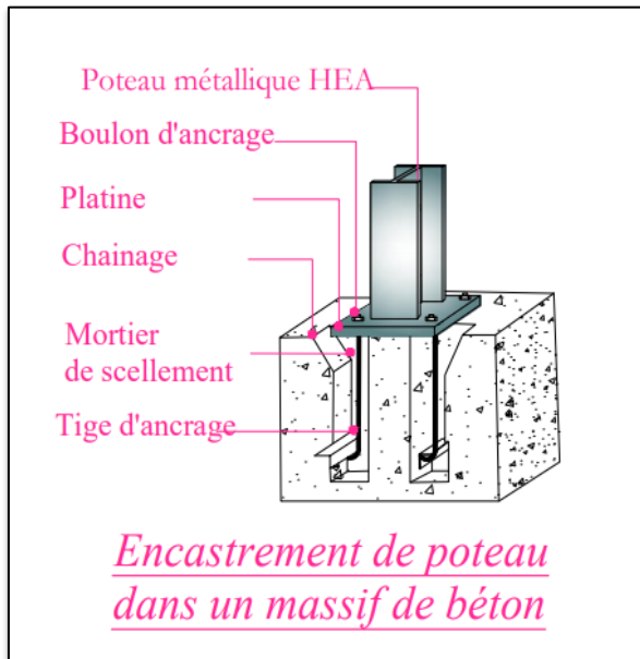
Figure 212 : détail assemblage poteau-fondations. Source : Autocad
