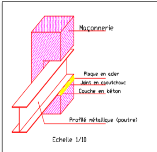
Figure 207 : détail assemblage poutre- poteau. Source : Autocad
