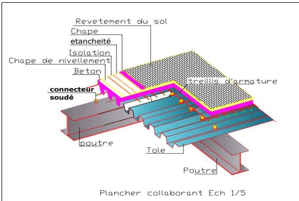
Figure 211 : Assemblage plancher et poutre
