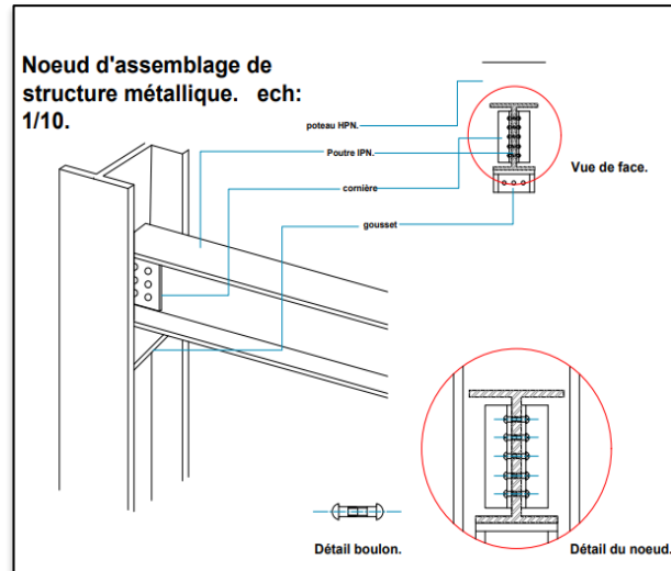
Figure 204 : détail assemblage poutre- poteau. Source : Autocad
