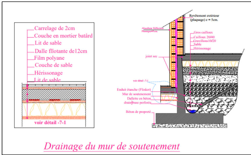
Figure 185 : Détail drainage du mur de soutènement.
