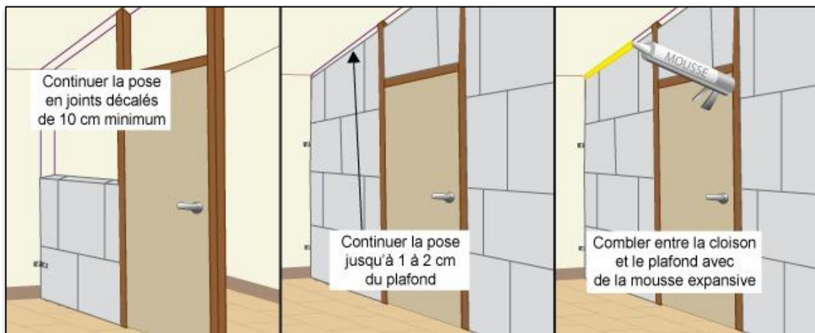
Figure 242 : Pose d'une cloison en béton cellulaire.
