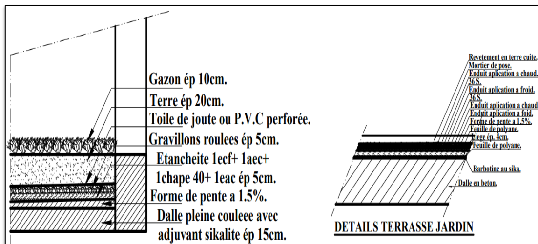
Figure 238 : Détail de la terrasse jardin Source : Autocad
