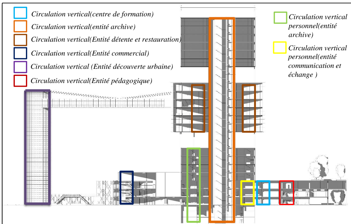
Figure 171 : Coupe illustrant la circulation vertical du projet Source : Revit
