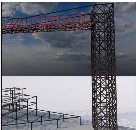
Figure 224 : Structure de l'ascenseur urbain. Source : Auteur
