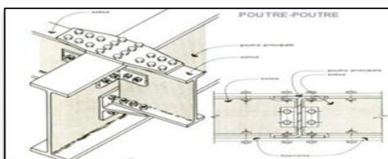
Figure 201 : détail assemblage poutre- poutre. Source : www.google .com
