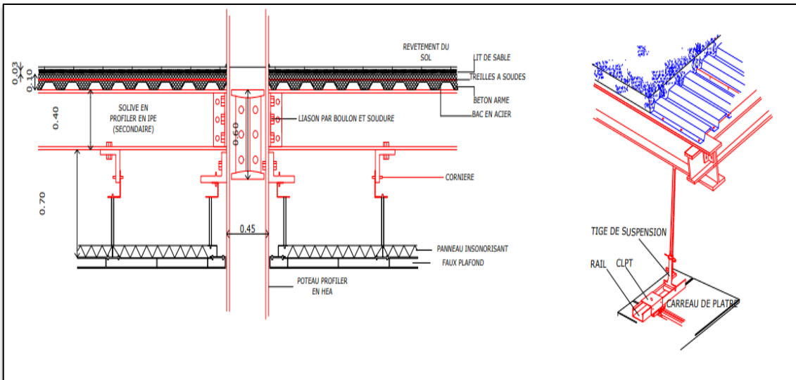
Figure 210 : détail assemblage poutre- poteau et plancher
