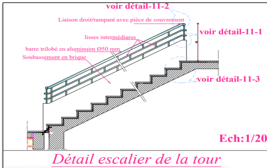
Figure 254 : Détail escalier en béton de la tour.
