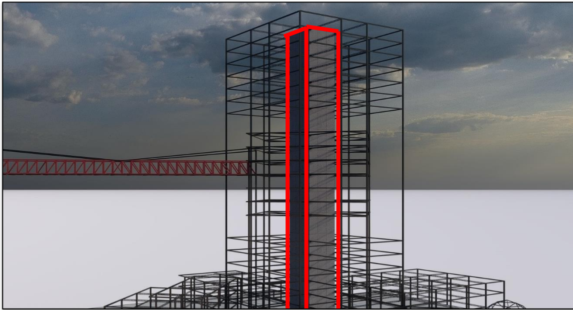
Figure 193 : Vue sur le noyau central du projet
