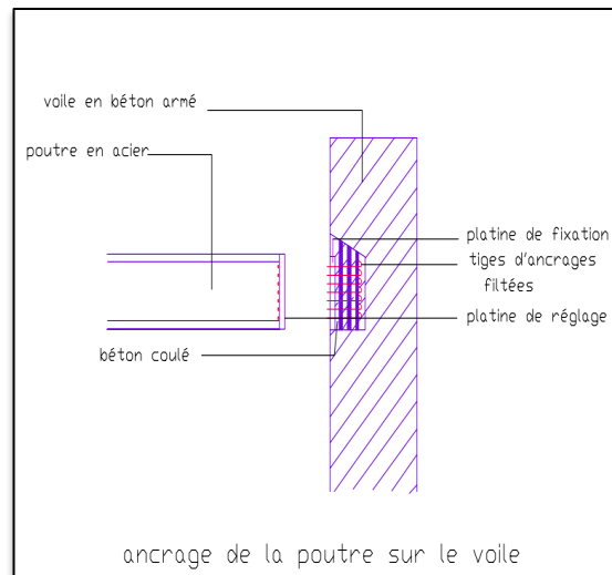
Figure 208 : détail assemblage poutre- poteau. Source : Autocad
