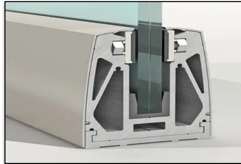
Figure 246 : fixation du vitrage de la cloison.
