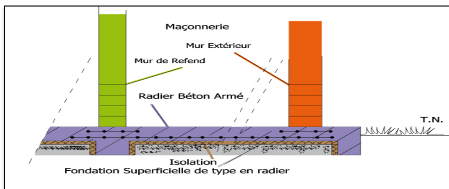
Figure 184 : Coupe qui montre un radier général.
