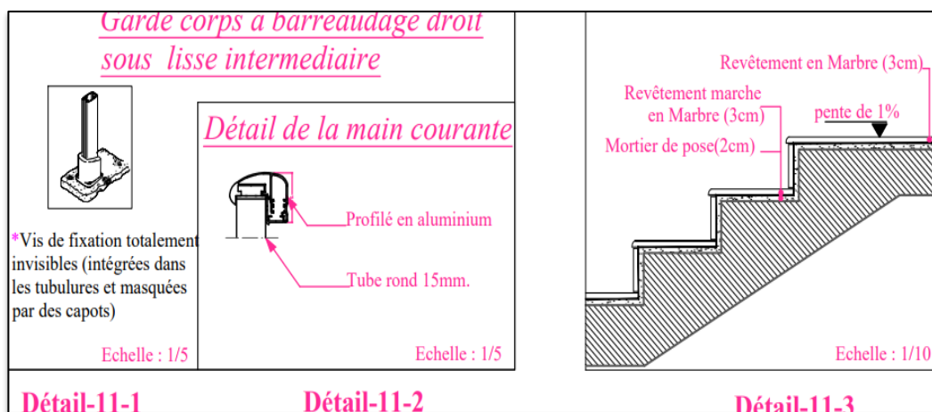
Figure 255 : Détail escalier en béton de la tour.
