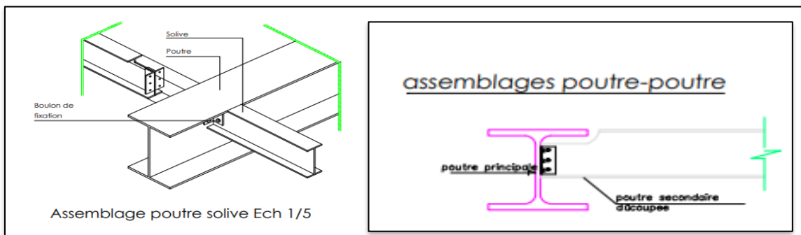
Figure 200 : détail assemblage poutre- poutre. Source : Autocad
