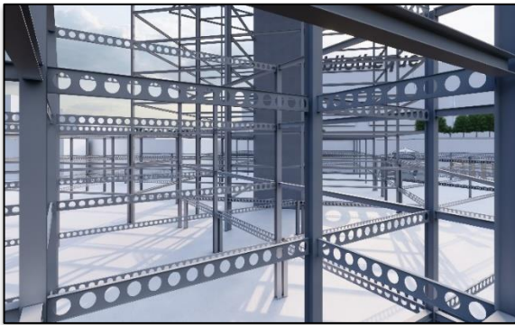
Figure 196: les poutres alvéolaires du projet. Source : Auteur
