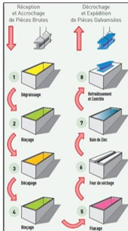
Figure 181 : les étapes du procédé de galvanisation
