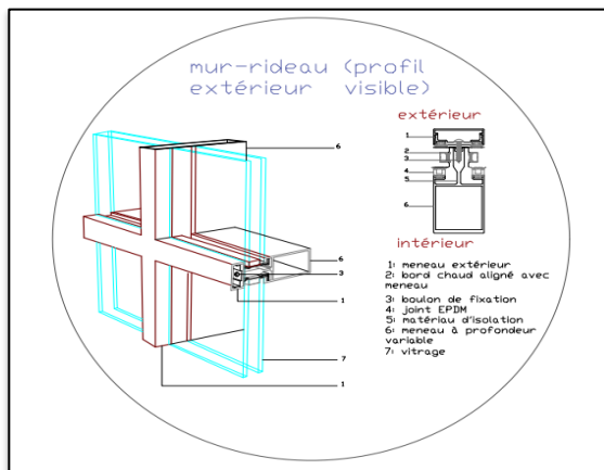
Figure 234 : Détail fixation du mur rideau.
