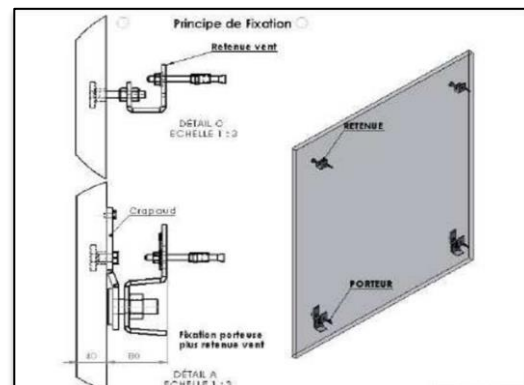
Figure 232 : fixation du ductal Source : http://www.fixinox.com
