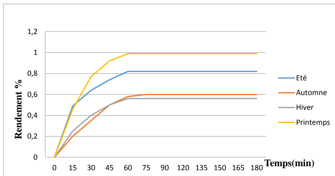
Figure 32 : Rendement en huile essentielle lors de l'hydro distillation des feuilles de Mentha spicata au cours de saison.
