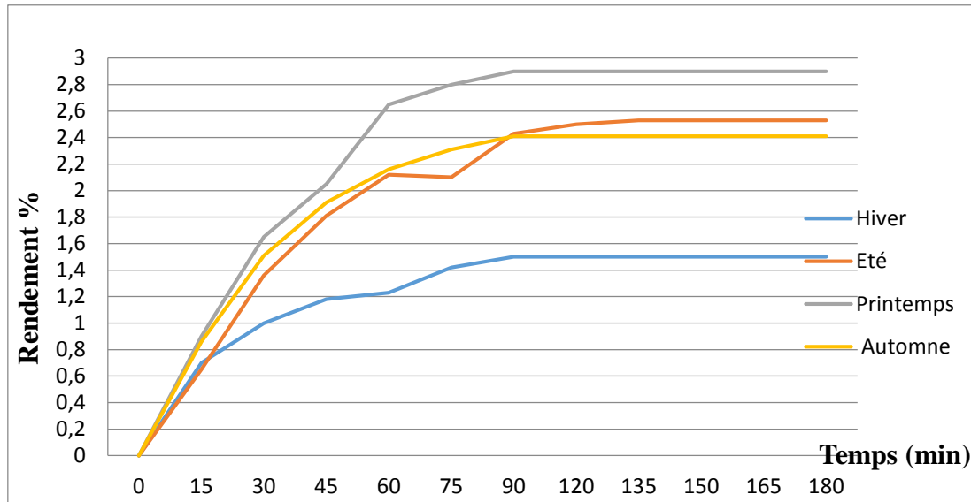
Figure 31 : Rendement en huile essentielle lors de l'hydro distillation des feuilles de Thymus vulgaris au cours de saison.
