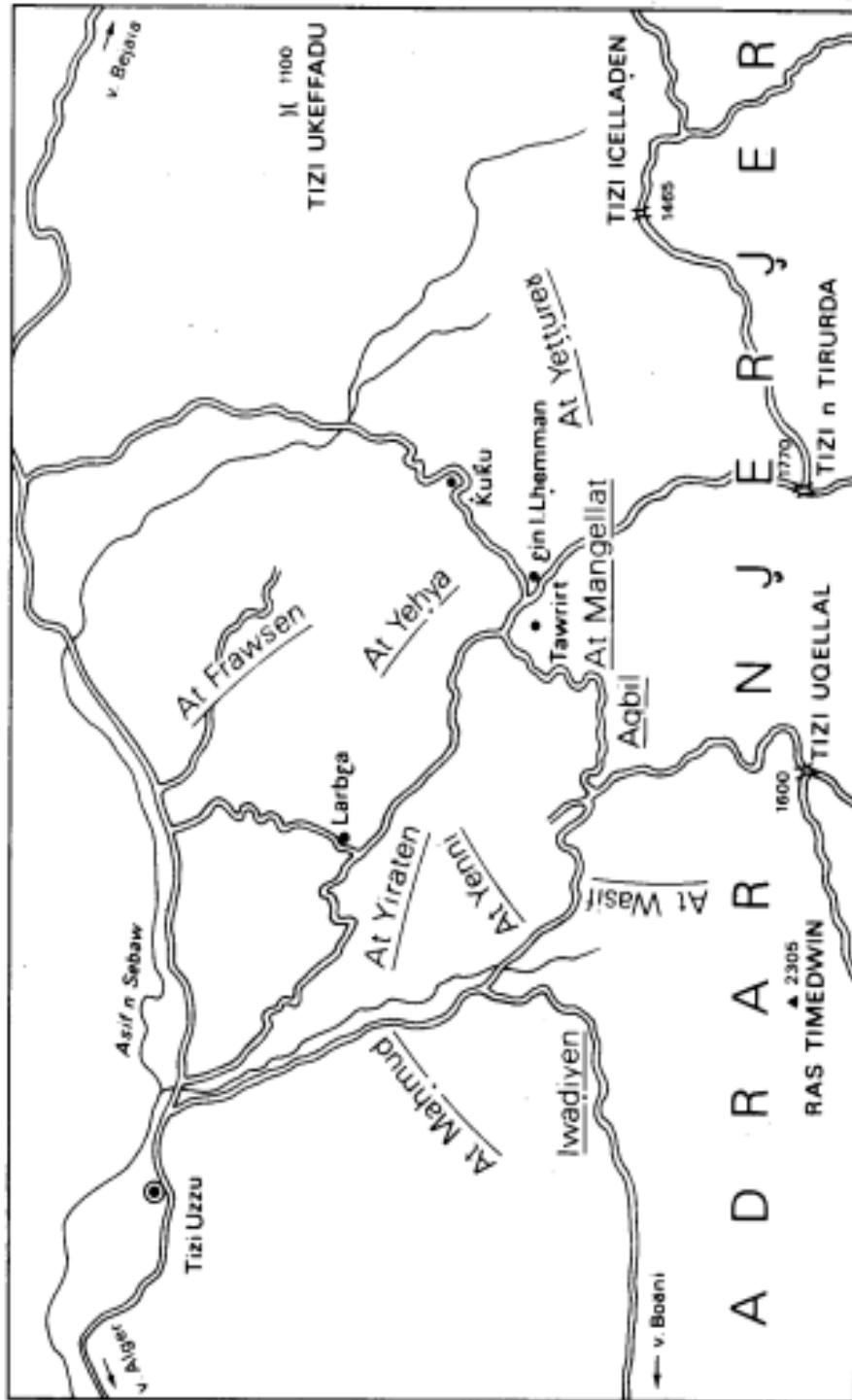
CARTE I. Les At Manguellat et leur environnement, à 130 km à l'Est d'El Jazaïr (Alger).
