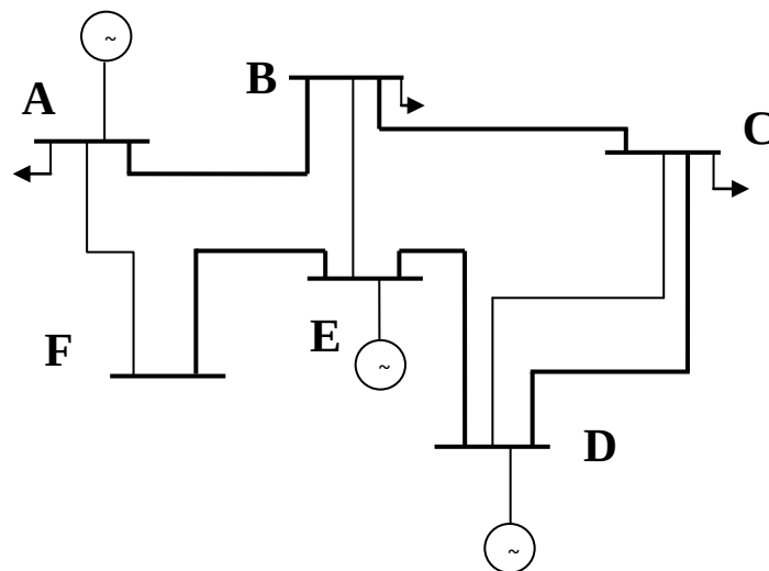
Figure I.2 : Réseau maillé [1]
