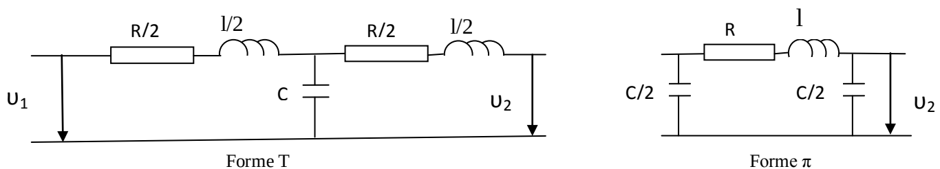
Figure II.2 : Schémas équivalents monophasés de forme T et \pi
