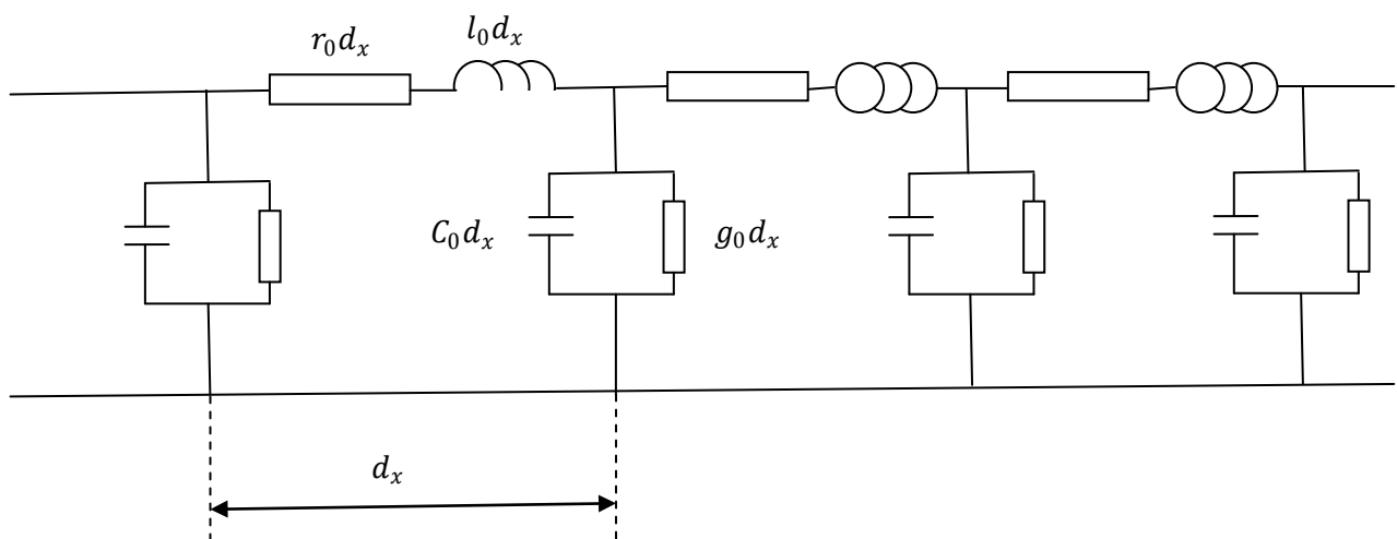
Figure II.1 : Schéma équivalent de la ligne triphasée en cascade.
