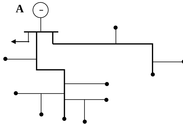
Figure I.5 : Réseau de distribution à structure radiale [1]
