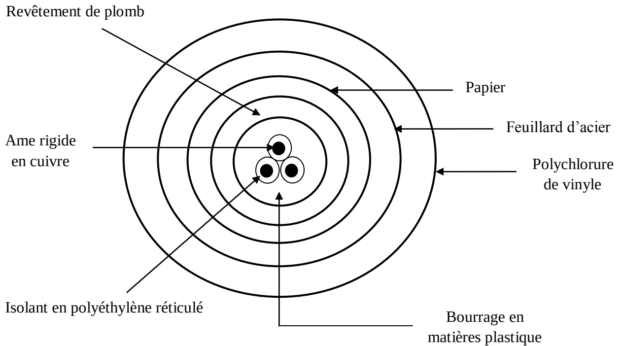
Figure I.8 : Vue en coupe d'un câble souterrain U 1000 RGPF V
