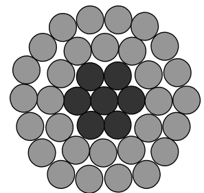
Figure III.9: câble Alu écroui
