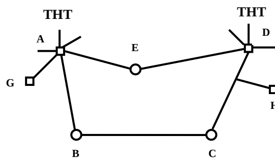
Figure I.3 : Structure bouclée
