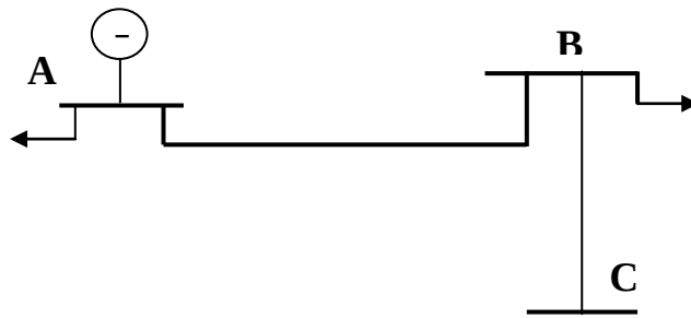
Figure I.6 : Réseau en antenne [1]
