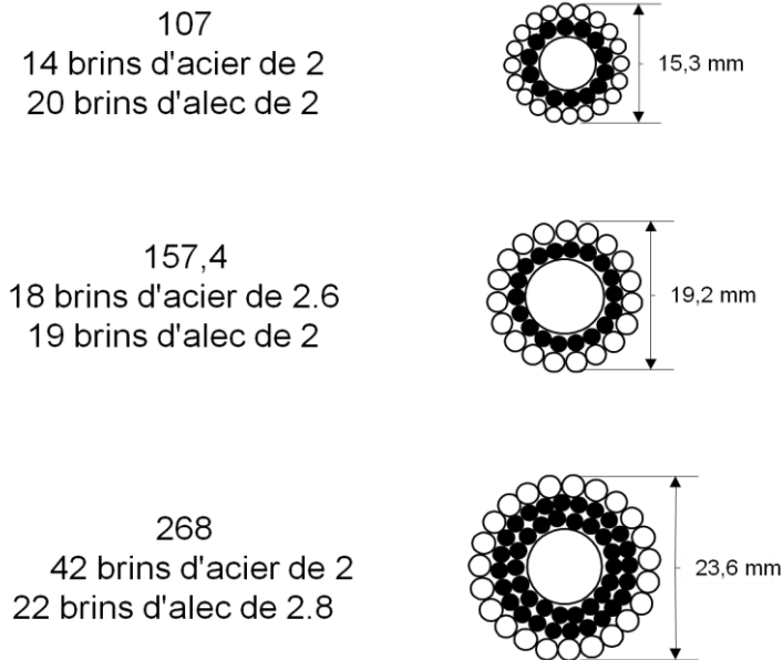
Figure III.13 : constitution de câble de garde
