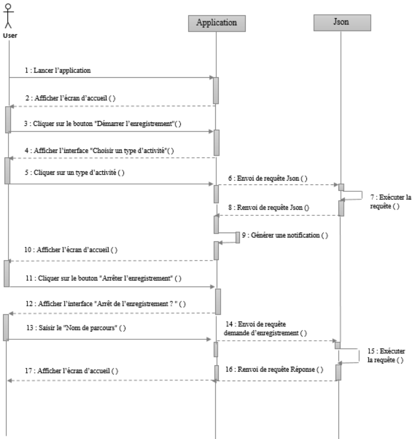
Figure 3.4. Diagramme de séquence de cas d'utilisation « Enregistrer un parcours ».
