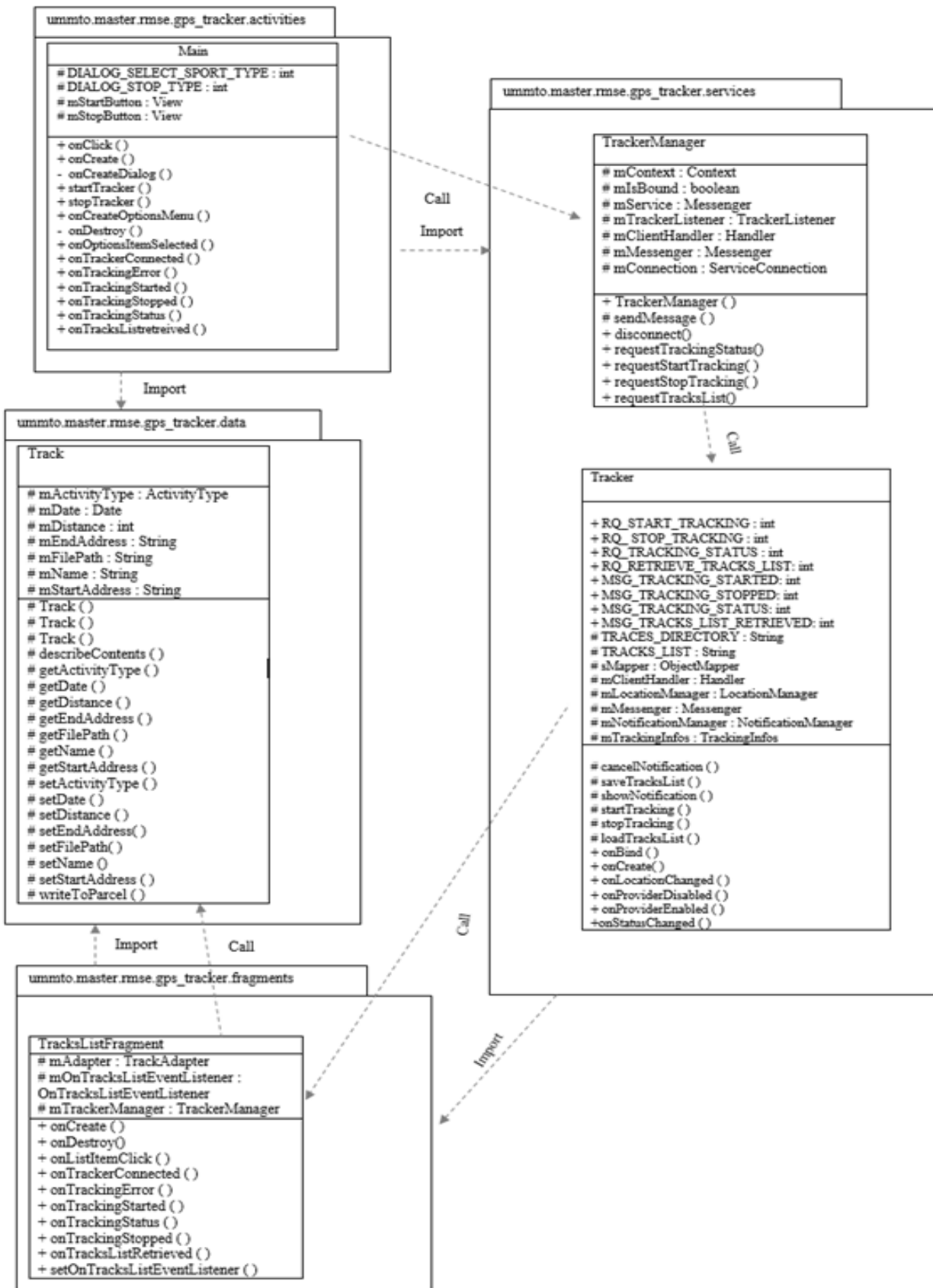
Figure 3.14 Diagramme de classe de cas d'utilisation : « Afficher les informations d'un parcours »
