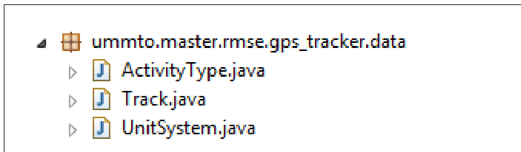
Figure 4.5. Package ummto.mastrer.rmse.gps_tracker.data
