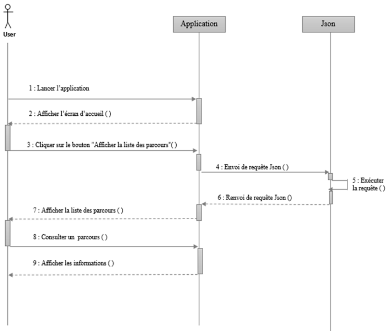
Figure 3.5. Diagramme de séquence de cas d'utilisation « Consulter les informations d'un parcours »
