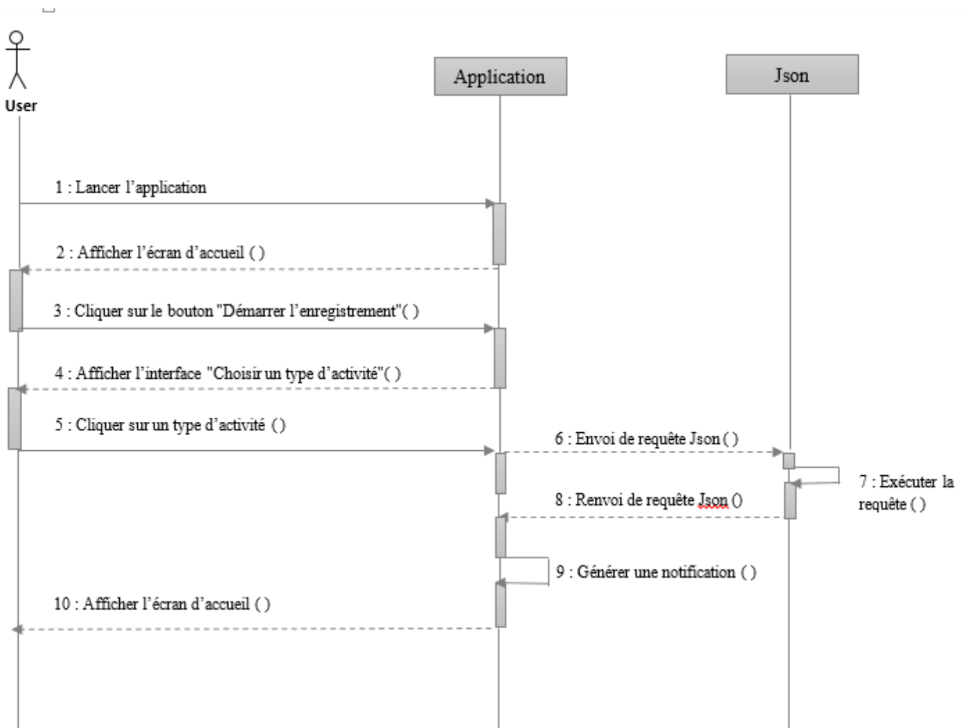
Figure 3.3. Diagramme de séquence de cas d'utilisation « Ajouter l'enregistrement d'un parcours ».
