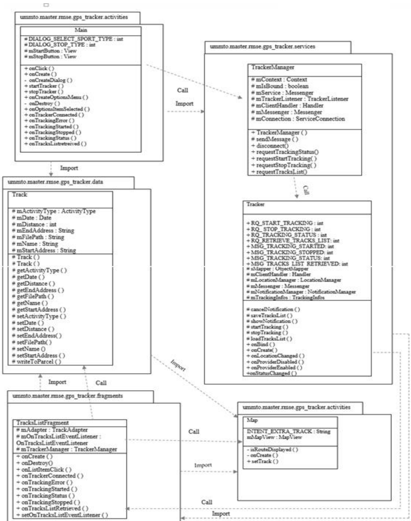
Figure 3.15 Diagramme de classe de cas d'utilisation : « Afficher un parcours sur une carte maps »
