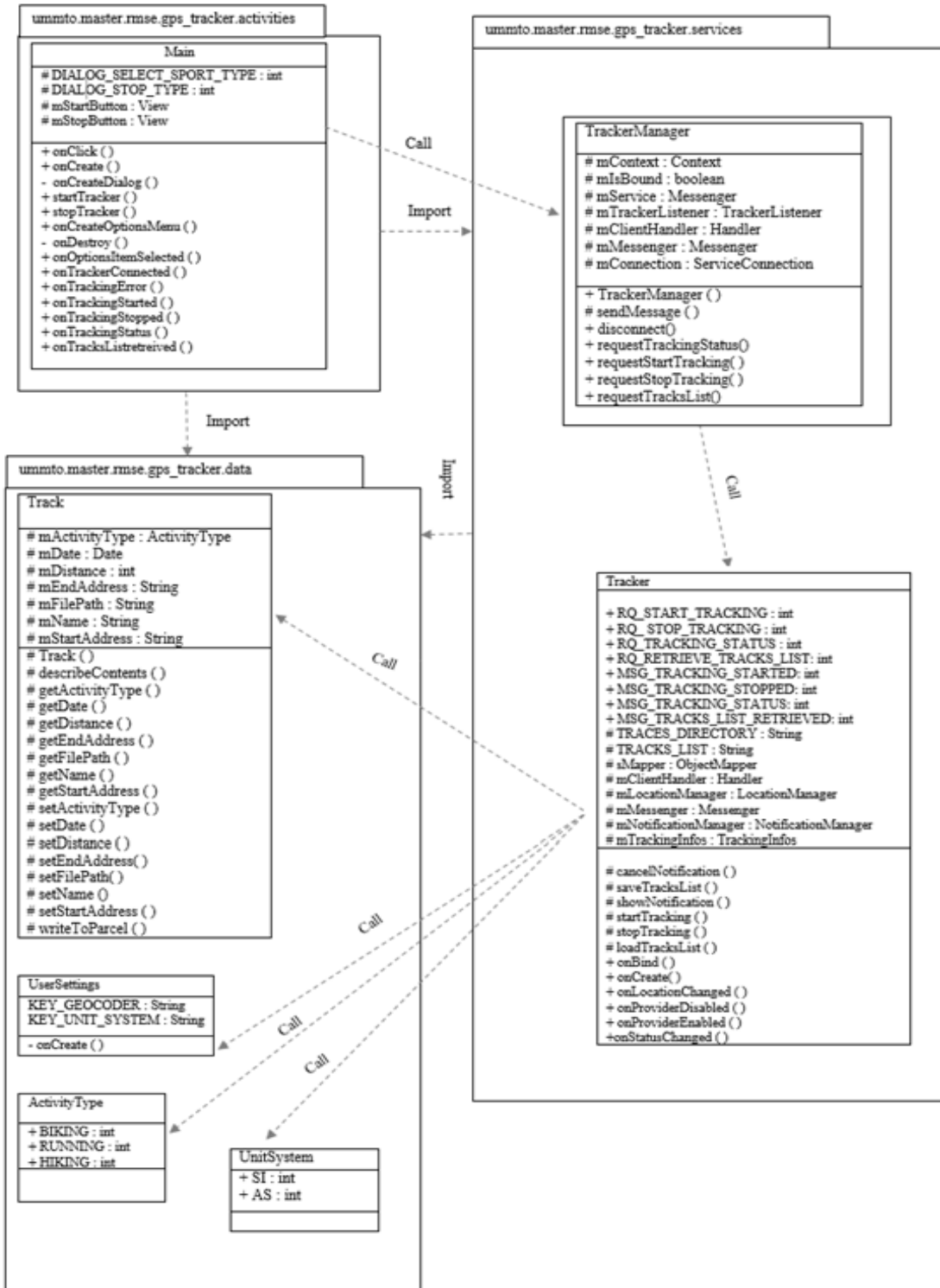
Figure 3.13. Diagramme de classes de cas d'utilisation: « Ajouter l'enregistrement d'un parcours »
