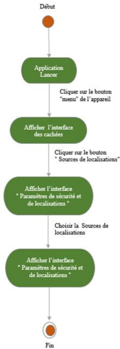
Figure 3.12. Diagramme d'activité de cas d'utilisation paramétrer l'application (Modifier la source de localisation)
