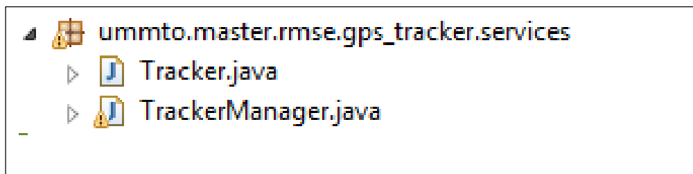
Figure 4.6. Package ummto.mastrer.rmse.gps_tracker.services
