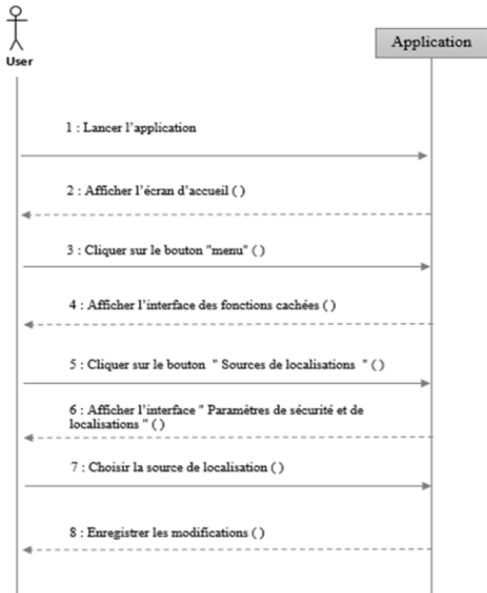
Figure 3.7 Diagramme de séquence de Cas d'utilisation « paramétrer l'application (Modifier la source de localisations) »
