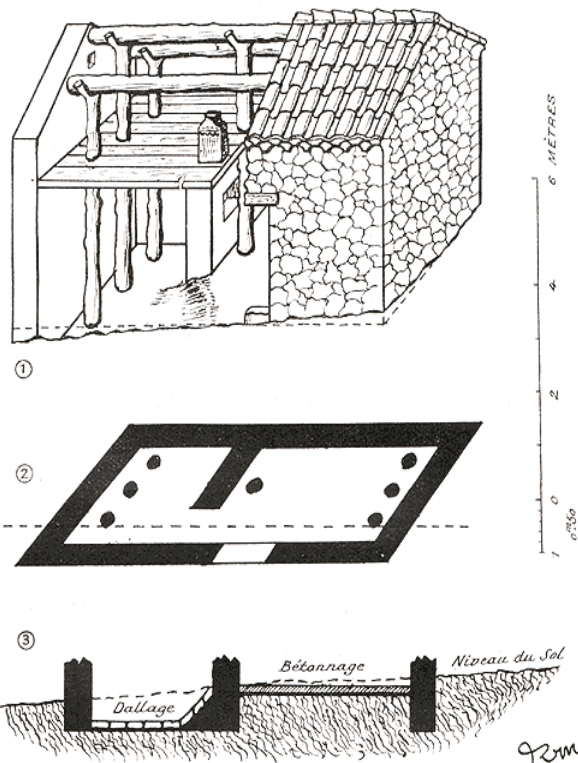
FIG. 1. — Vue cavalière, plan et coupe d'une maison kabyle.
