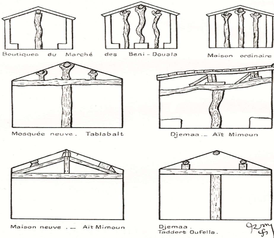
FIG. 5. — Charpentes kabyles.
