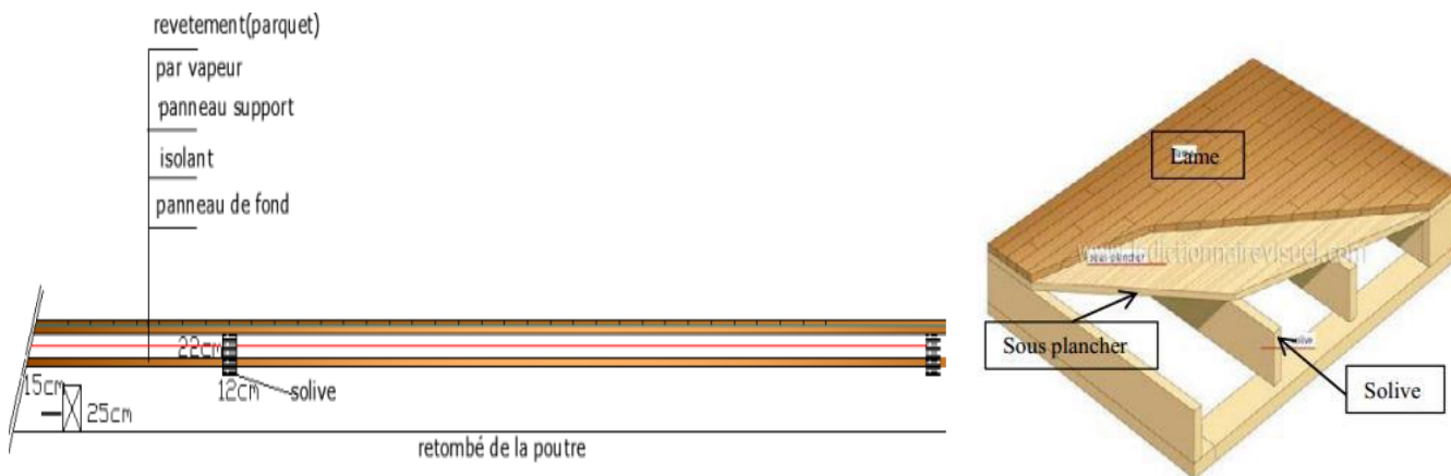
Figure(159) : Plancher en bois
