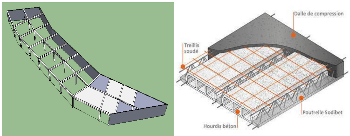
Figure(160) : structure de parking source :établis par Auteurs Figure (161): Plancher en corps creux Source: Google image/plancher
