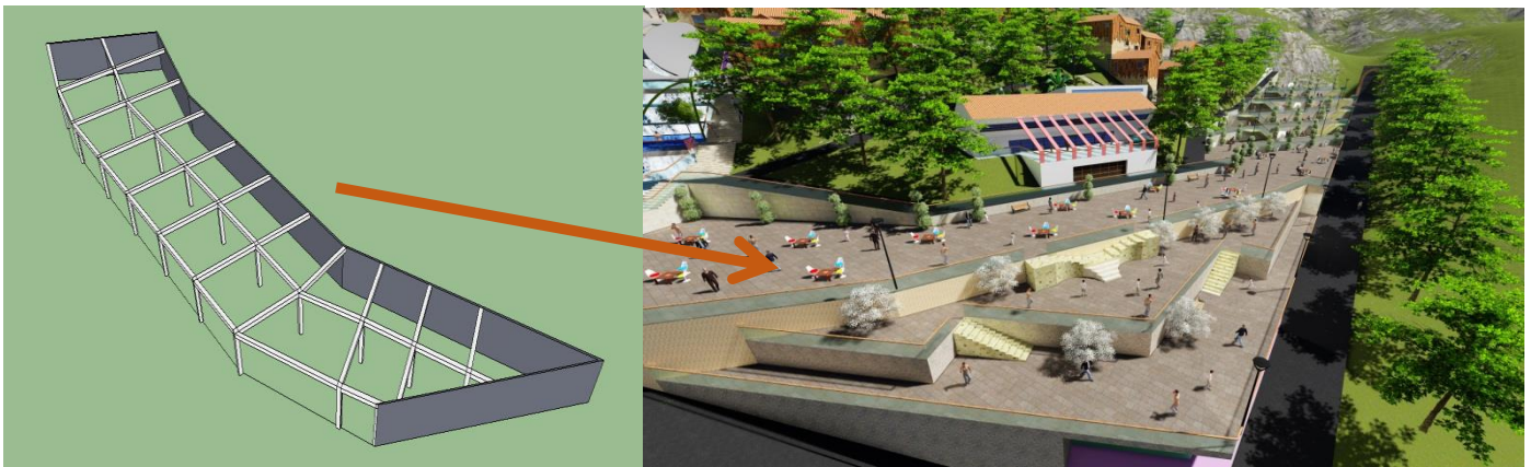
Figure(156) : structure de parking source : établis par Auteurs
