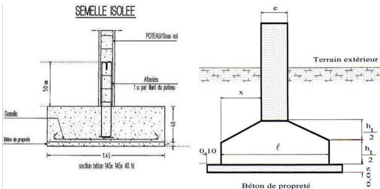
Figure(155) : Semelle isolée en coupe Source:Google image/semelle isolée
