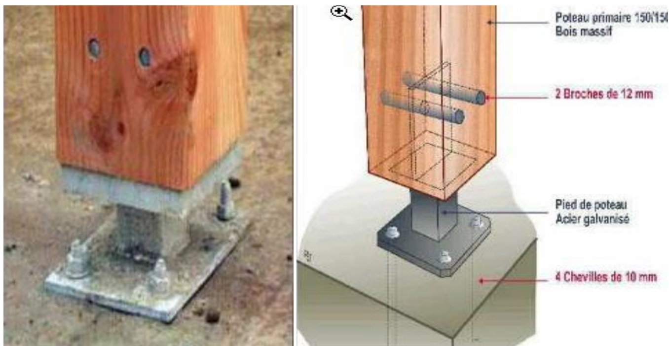
Figure(162) : Ancrage de poteau en bois dans la fondation Source:PDF/ Constructiondemaïsons à ossaturebois «Thierry Paradis»
