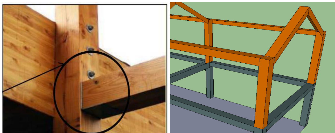
Figure(163) : Assemblage poteau-poutre Source:PDF/ Constructiondemaïsons à ossaturebois «Thierry Paradis»
