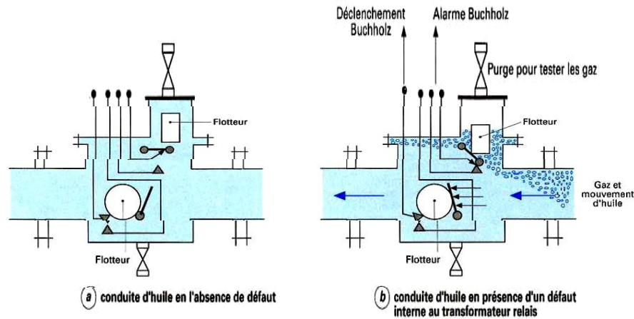
Figure (III-6): Principe de fonctionnement de relais Buchholz
