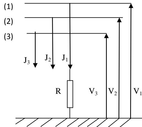
Figure (II-2) : court-circuit monophasé
