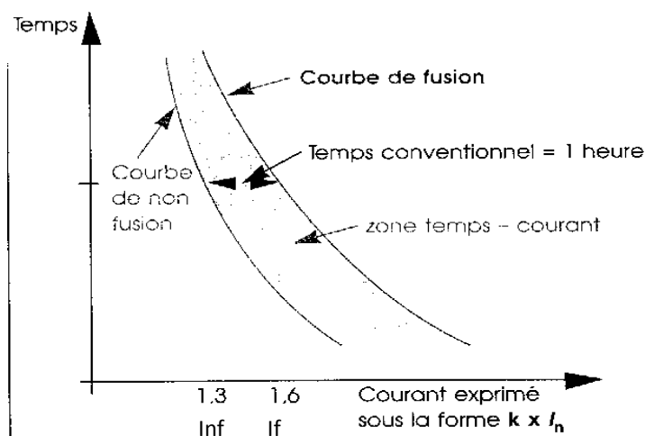
Figure (III-3) : courbe caractéristique d'un fusible
