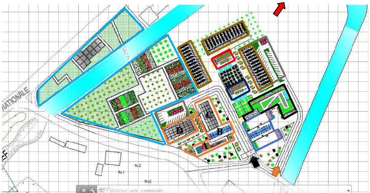
Figure VI.4 : Organisation de plan de masse Source : Auteurs
