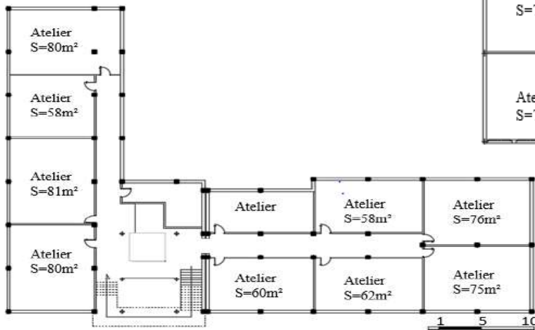
Figure III.3.34 : Plan RDC du bloc A
