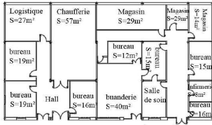
FigureIII.3.48 : Plan type d'un bloc résidentiel
