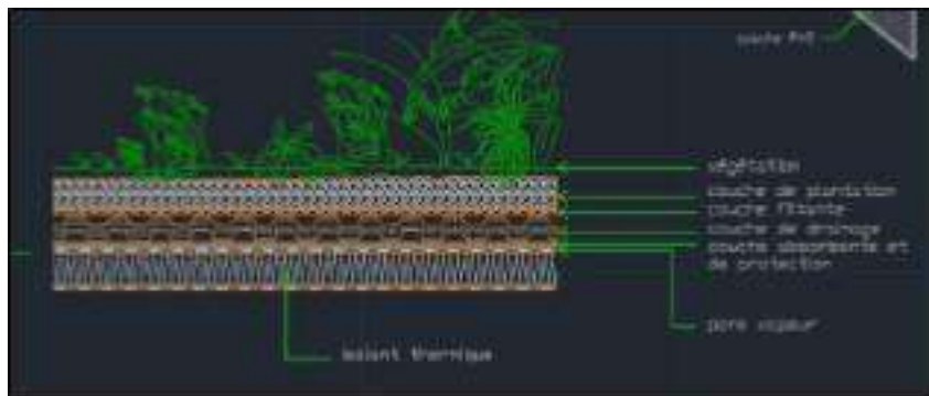
Figure VI.16: Détail terrasse végétale
