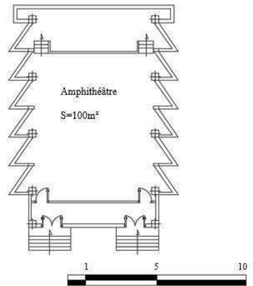
FigureIII.3.38 : Plan de l'amphithéâtre Source :auteurs
