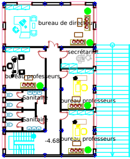
plan sous sol
