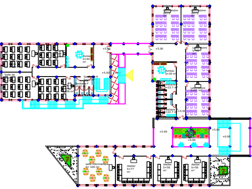
plan de 1ère étage
