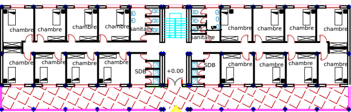
plan de rez de chaussée
