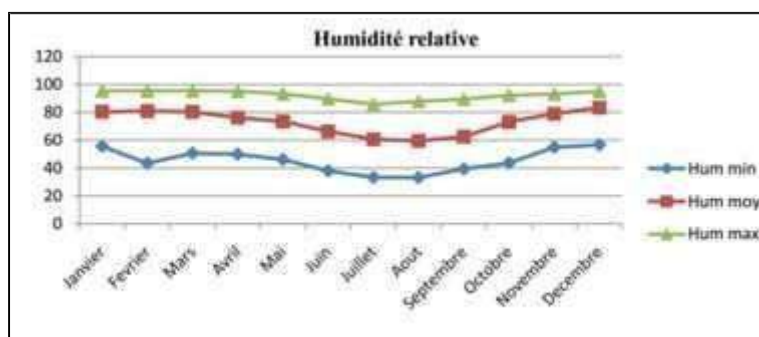
Figure III.2.26: Diagramme des valeurs de l'humidité annuelle à Tizi-Ouzou Source : Diagramme élaboré d'après les données climatiques relevées par la station ONM de Boukhalfa, 2008/2017)
