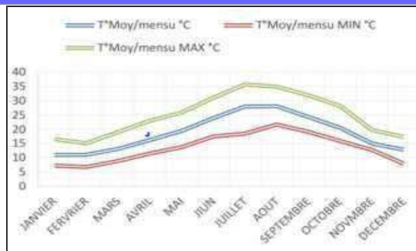
Figure III.2.25: Diagramme des valeurs des températures moyennes mensuelles. Source : Diagramme élaboré d'après les données climatiques relevées par la station ONM de Boukhalfa, 2008/2017)
