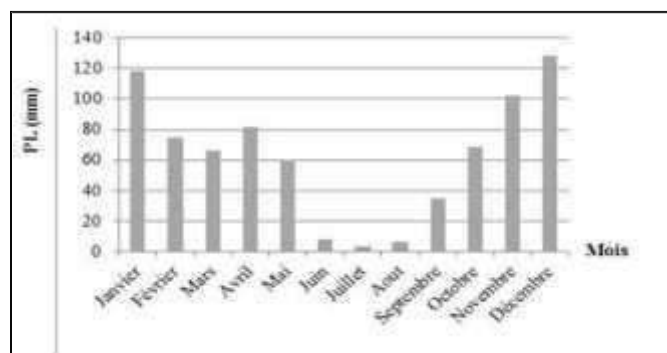
FigureIII.2.28: Histogramme des précipitations moyennes annuelles à Tizi-Ouzou.
