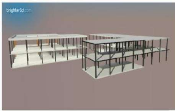
Figure VI.12 : Modélisation de la structure de l'administration et la bibliothèque.
