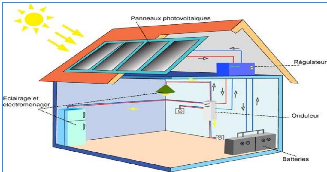
Fig. III.3 : Schématisation de l'énergie solaire non connectée au réseau (Off Grid)
