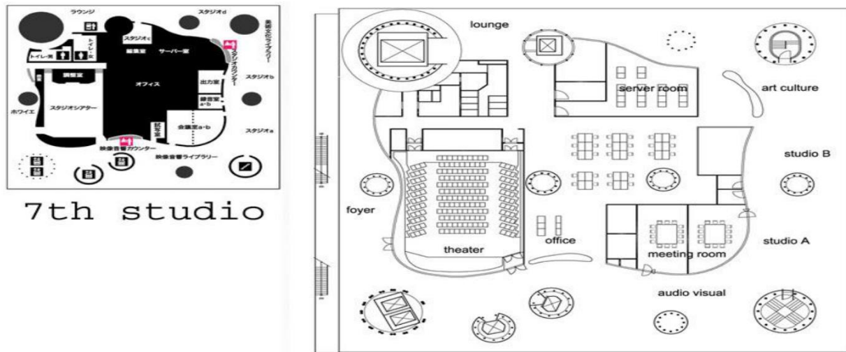
Fig 52 : Plan de 7 ème niveau de la médiathèque de Sendai
