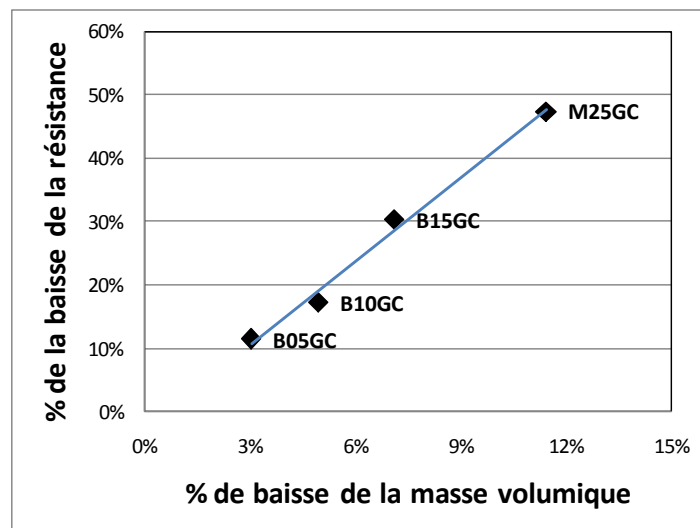
Figure III.4. % de baisse de la Rc à 28 jours en fonction du % de baisse de la masse volumique
