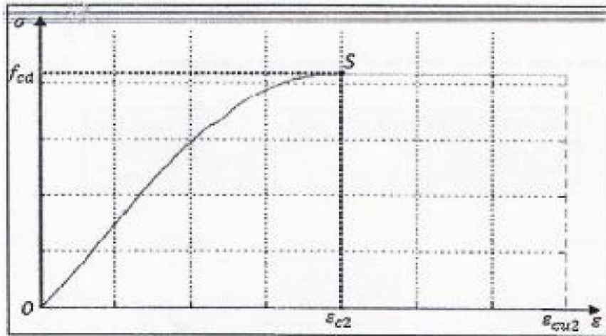
Figure I.16: Diagramme parabolique-rectangle du béton en compression [18].
