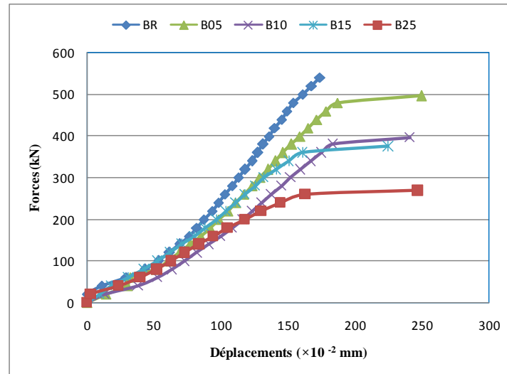
Figure III.8 : superposition des courbes de force fonction des déplacements enregistrés.
