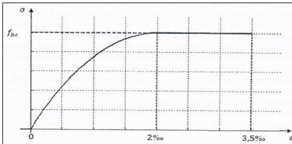
Figure I.15 : Loi parabole-Rectangle du béton en compression [17].
