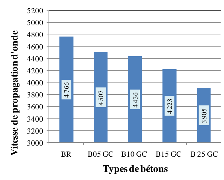
Figure III.5 : Histogramme des vitesses à l'ultrason au 28ème jour.
