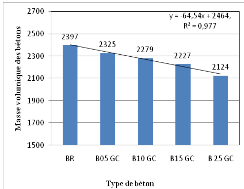
Figure III.1. Masse volumique des bétons en fonction du pourcentage en GC
