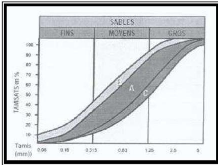
Figure 1.8. Fuseaux préférentiels pour la granularité des sables pour béton selon la méthode de Dreux Gorisse [4].
