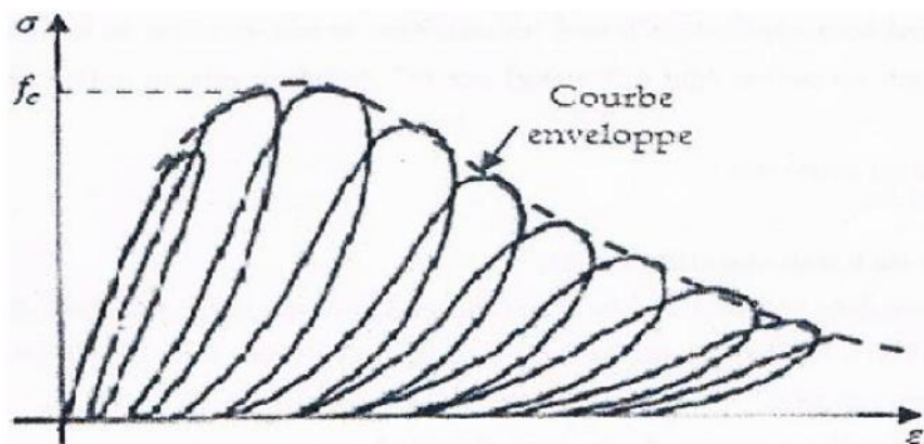
Figure I.14: Comportement cyclique du béton en compression simple, [15]
