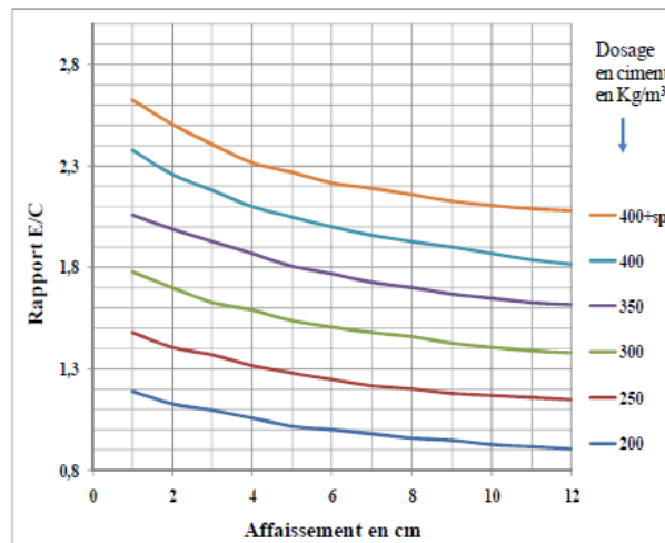
Figure I.7. Dosage en ciment en fonction de rapport E/C et de l'affaissement au cône d'Abrams [4]
