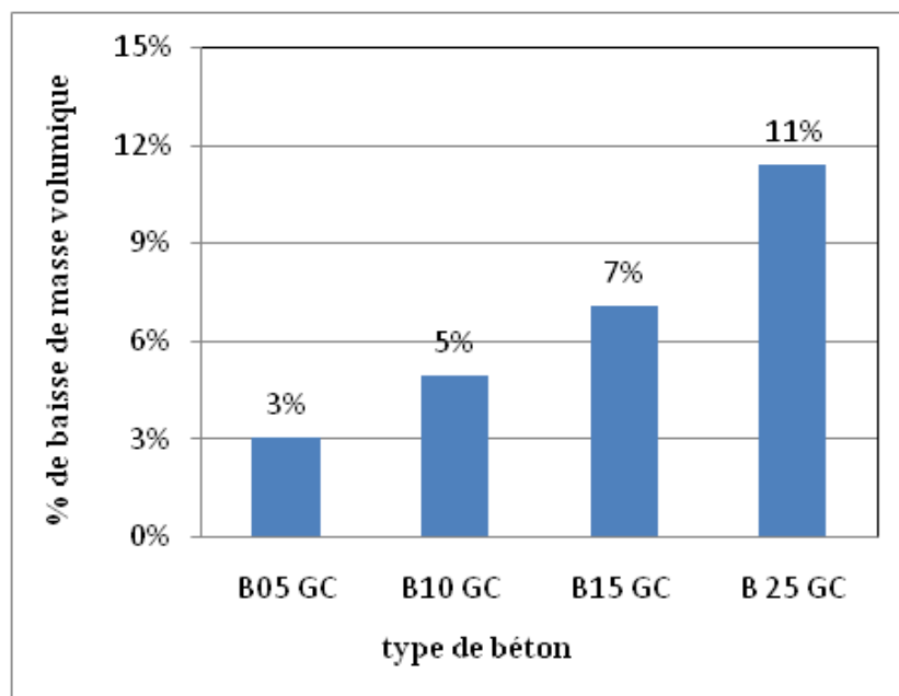
Figure III.2. Pourcentage de baisse des masses volumiques des bétons en fonction du % en GC
