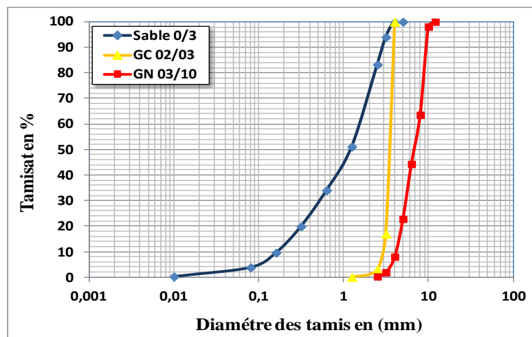
Figure II.3 Courbe granulométriques du sable 0/3, gravier 3/8 et des granulats en caoutchouc
