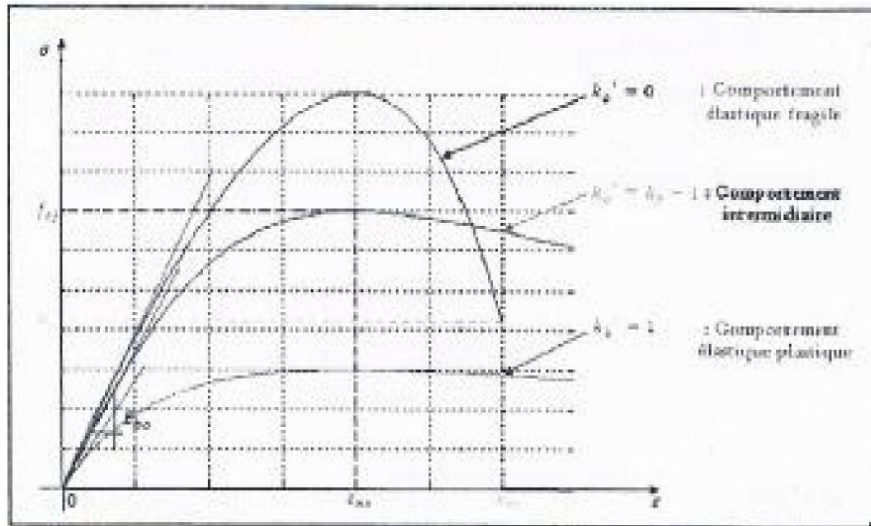
Figure I.17: Comportement du béton en compression selon Sargin(1971) .
