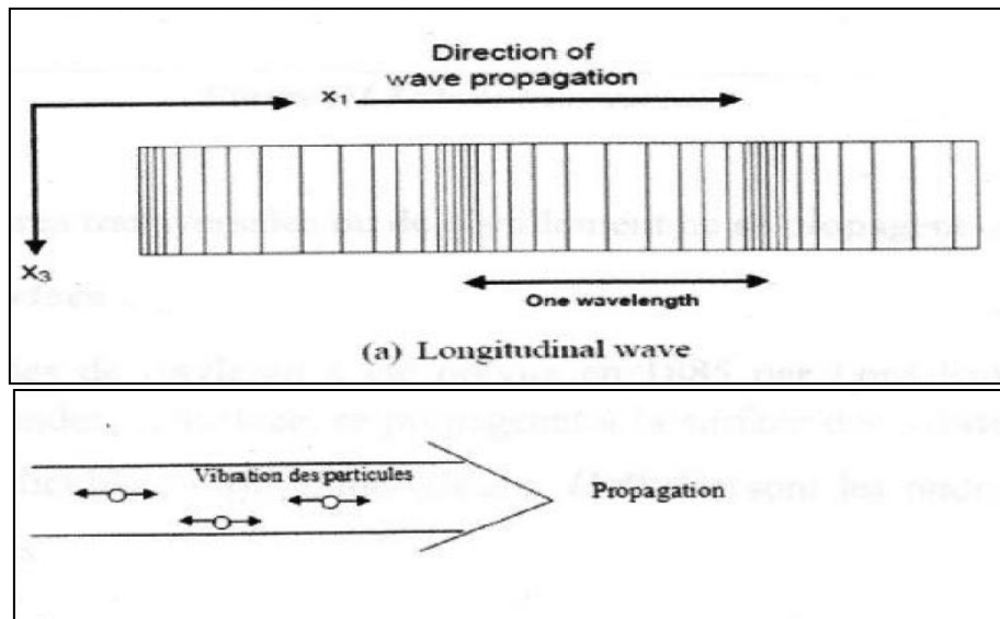
Figure I.15 Ondes longitudinales
