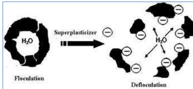
Figure I.4. Défloculation du ciment par l'action dispersante des superplastifiants.
