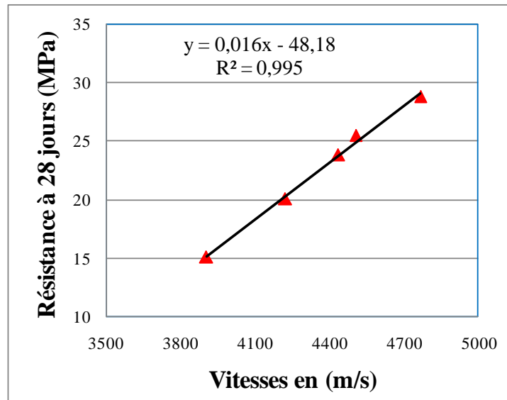
Figure III.6 : Corrélation entre les résistances à la compression et les vitesses à l'ultrason (à 28 jours).
