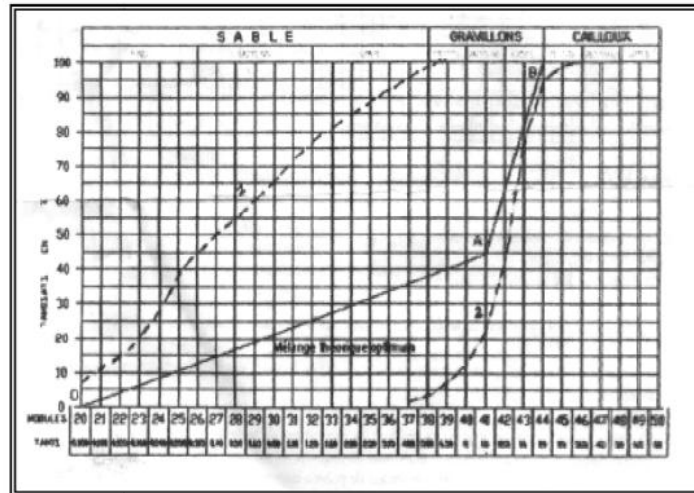
Figure 1.9. Courbe du mélange optimum selon la méthode de Dreux-Gorisse [4]
