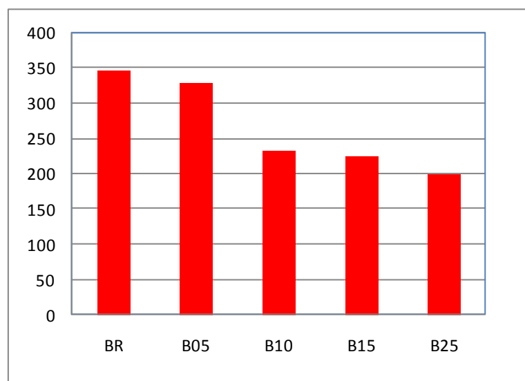
Figure III.9 : histogramme représentatif des modules de déplacements (kN/mm)
