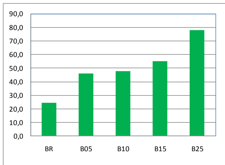
Figure III.10 : histogramme représentatif des déplacements ductiles ( \times 10^{-2} mm)
