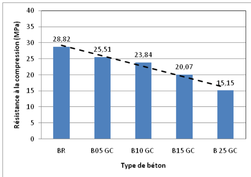
Figure III.3. Histogramme des résistances à la compression à 28 jours des bétons
