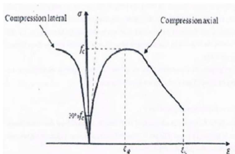
Figure I.13: comportement du béton en compression [14]
