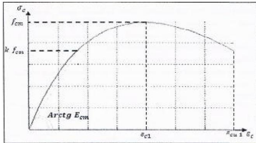
Figure I.16 : Diagramme non linéaire du béton en compression EUROCODE2 .
