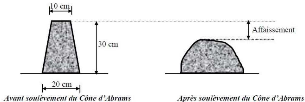
Figure I.6. Courbes illustratives de l'essai d'affaissement au cône d'Abrams.
