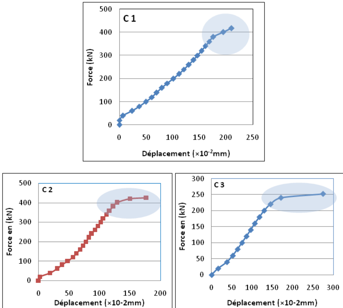
Figure III.7 : Exemples de courbes de force (kN) fonction des déplacements (mm) enregistrés.
