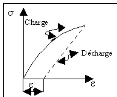
Figure I.12: diagramme de déformation plastique.
