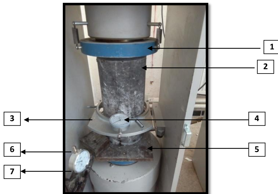
- Figure II.8. : Essai de déformation
