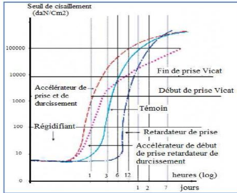
Figure 1.5. Courbes d'évolution du seuil de cisaillement (début de prise) en fonction de la présence d'un accélérateur ou d'un retardateur de prise [10].
