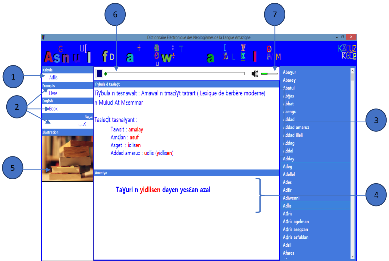
Figure 07.2 : Résultat de la recherche du mot « Adlis ».
