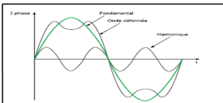
Figure I.1: signal déformé
