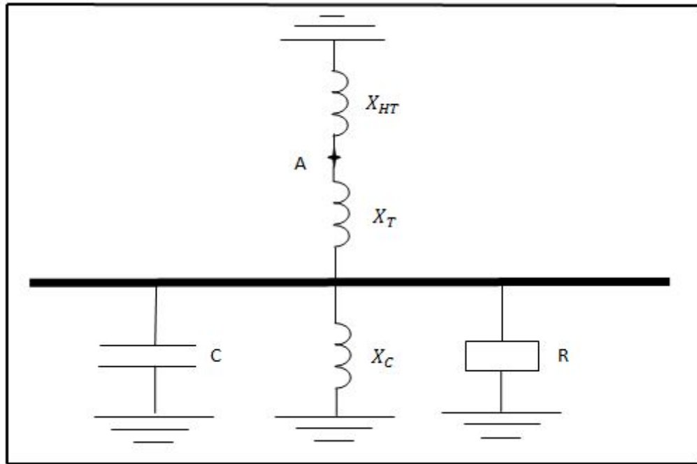
Figure II.4 : Exemple d'un réseau
