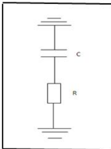
Figure II .13 : Filtre amorti du premier ordre
