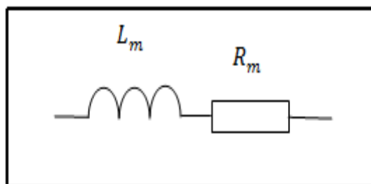
Figure II.22: modèle d'un moteur
