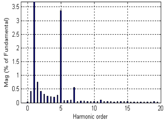
Figure III.3 : Forme d'onde et spectre de la tension au jeu de barres (03-MILL-1)
