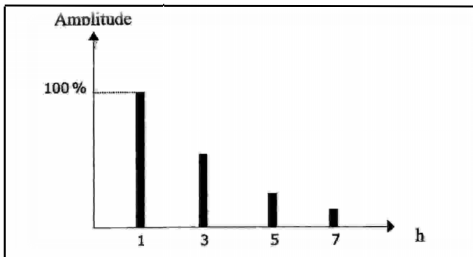
Figure 1.2 : Représentation spectrale d'un signal déformé.
