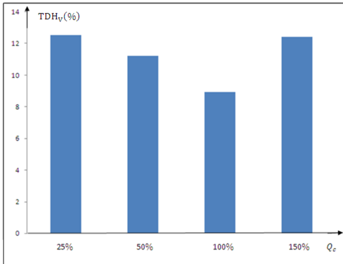
Figure III.13 : TDH_V (%) en fonction de Q_c
