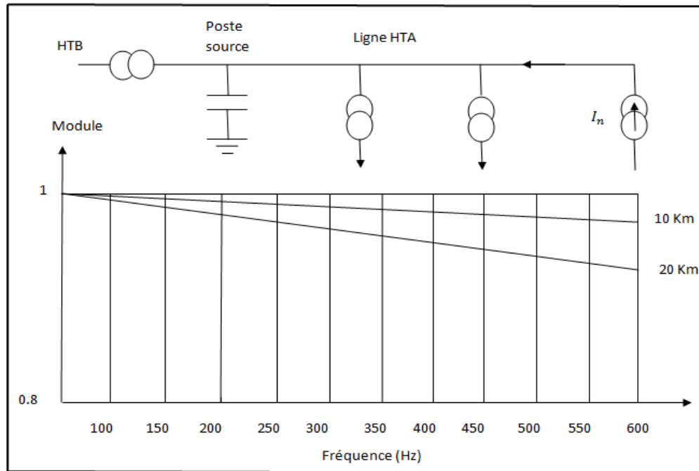
Figure II.3 : Atténuation du courant sur un réseau en fonction de la fréquence
