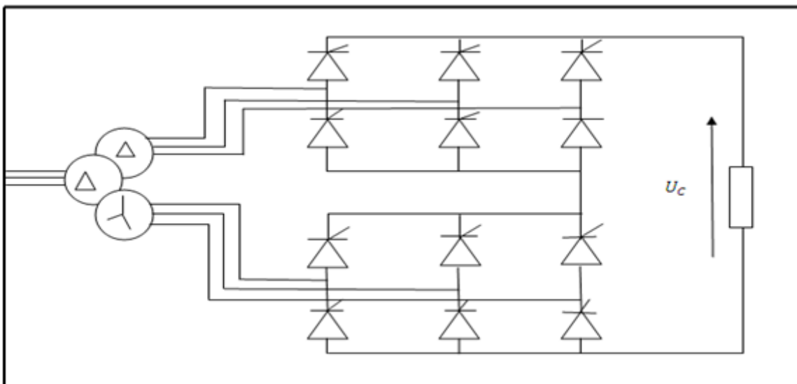
Figure II .27 : Montage dodécaphasé
