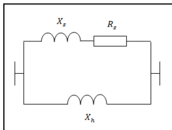
Figure II.23 : modèle de CIGRE
