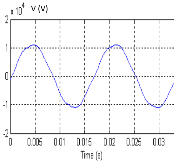
Figure III.3 : Forme d'onde et spectre de la tension au jeu de barres (03-MILL-1)
