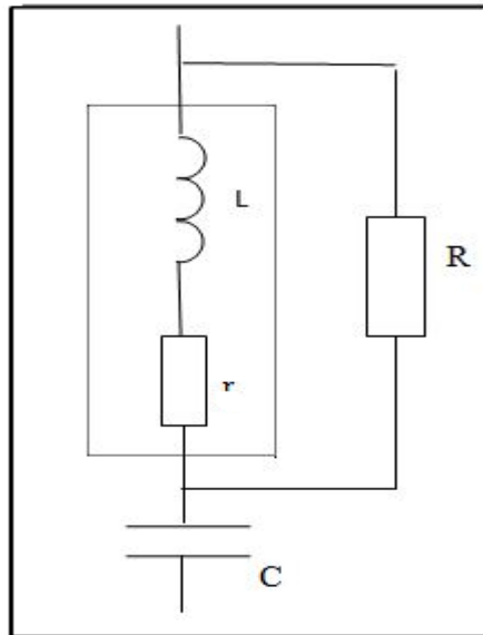
Figure II.12: Structure d'un filtre amorti
